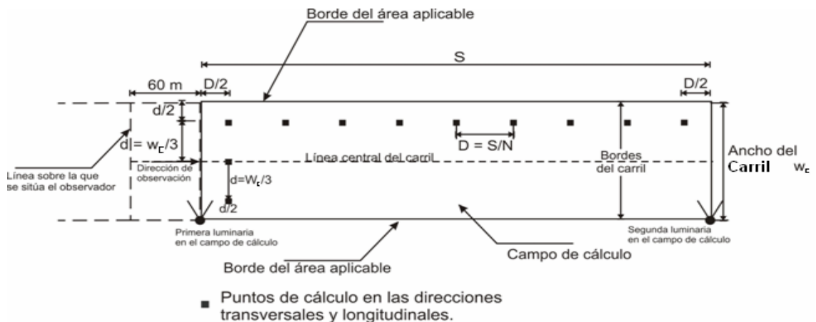
Figura 530.3.6 b) Posición de los puntos de cálculo en un carril.
