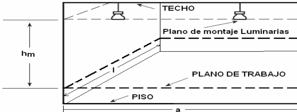
Figura 430.1. a) Distancias y cavidades para aplicación del método del Coeficiente de local
