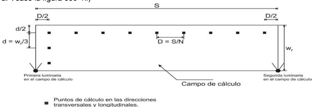
Figura 530.1.I) Puntos de cálculo para la iluminación
