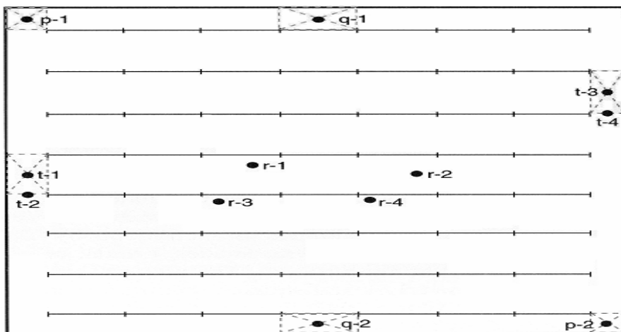
Figura 490.1 d) Puntos de medición de iluminancia en la cuadrícula de un local con dos o más filas de luminarias
