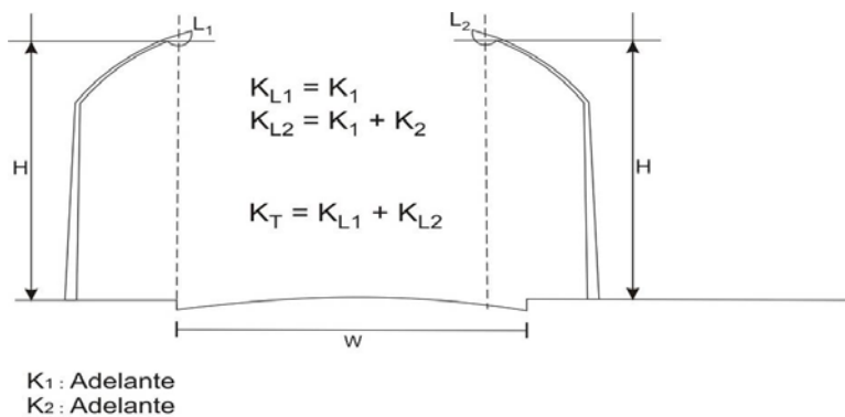
Figura 520-1.j) Localización bilateral alternada (zig-zag ó tres bolillos)
