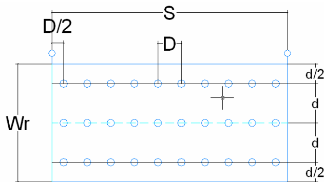
Figura 530-4.1 Malla de medición para Iluminancia
