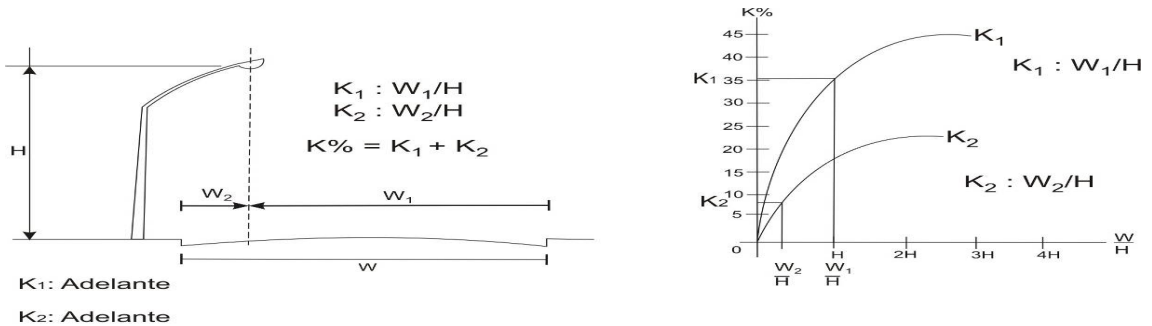
Figura 530-1.g) Luminaria sobre la calzada
