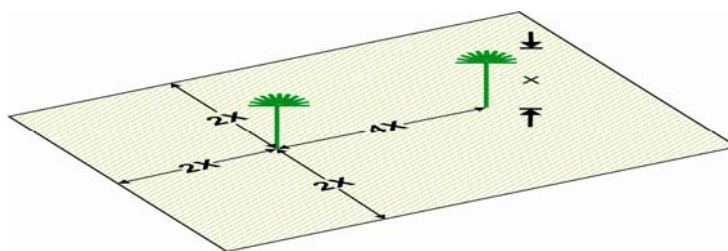
Figura 550.1 a) Ubicación de mástiles en el centro del área
