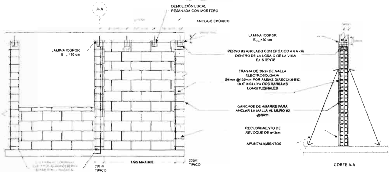
Figura A.3 -15 Dilatación de muros existentes.
